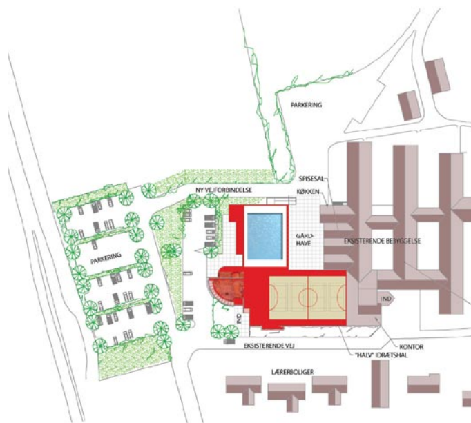
Oversigtsplan for udkastet til de nye udvidelser
