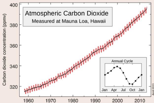
Keelings kurver. (Kilde: Manua Loa observatoriet)
